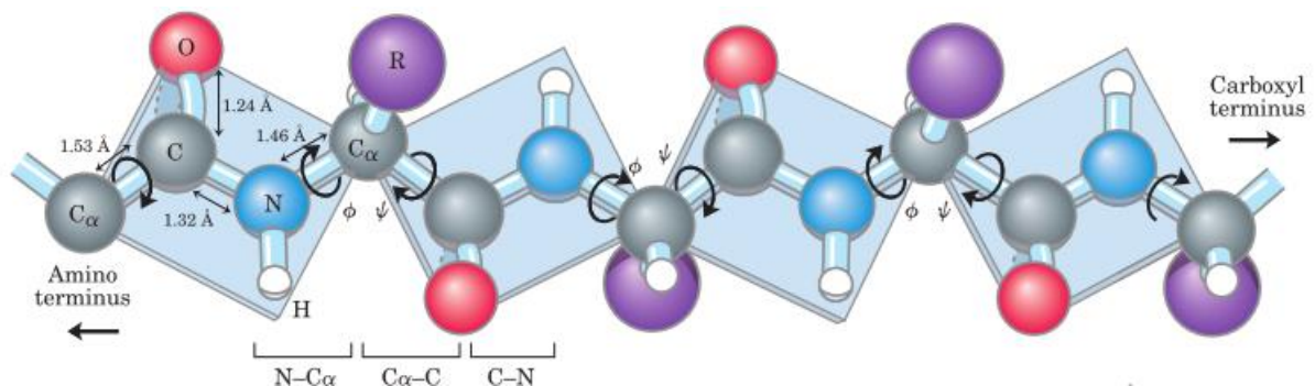
Figura 4 – Esquema das conexões entre os aminoácidos e ângulos φ e ψ.
