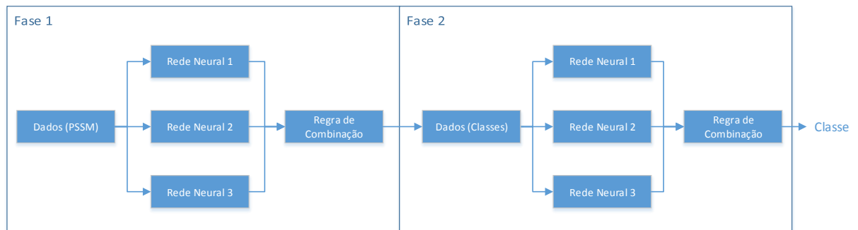
Figura 13. Arquitetura do preditor desenvolvido.
