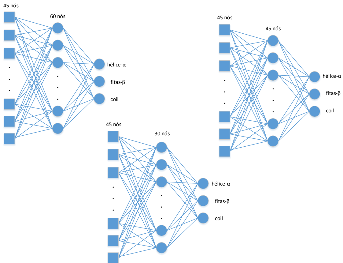
Figura 15 – Estrutura da fase estrutura-estrutura do preditor proposto.
