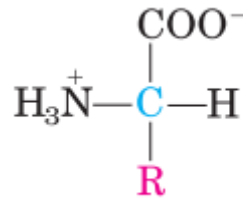
Figura 3 – Esquema geral de um aminoácido.
